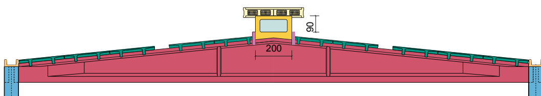
trave doppia pendenza con torrino
