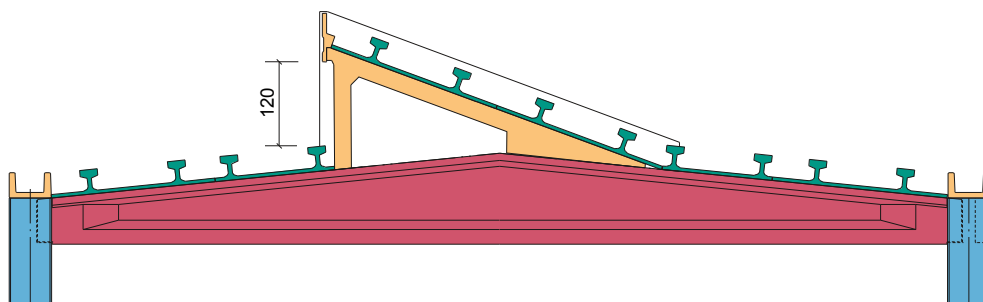
trave doppia pendenza con shed
