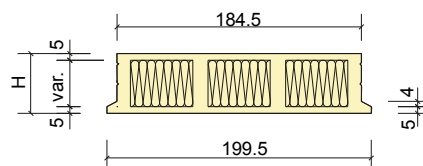
sezione
