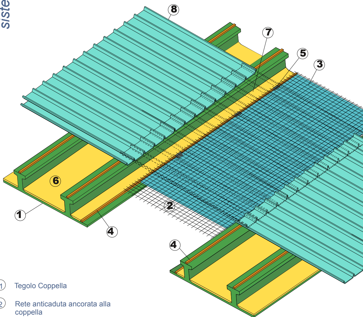
Montaggio lucernario
