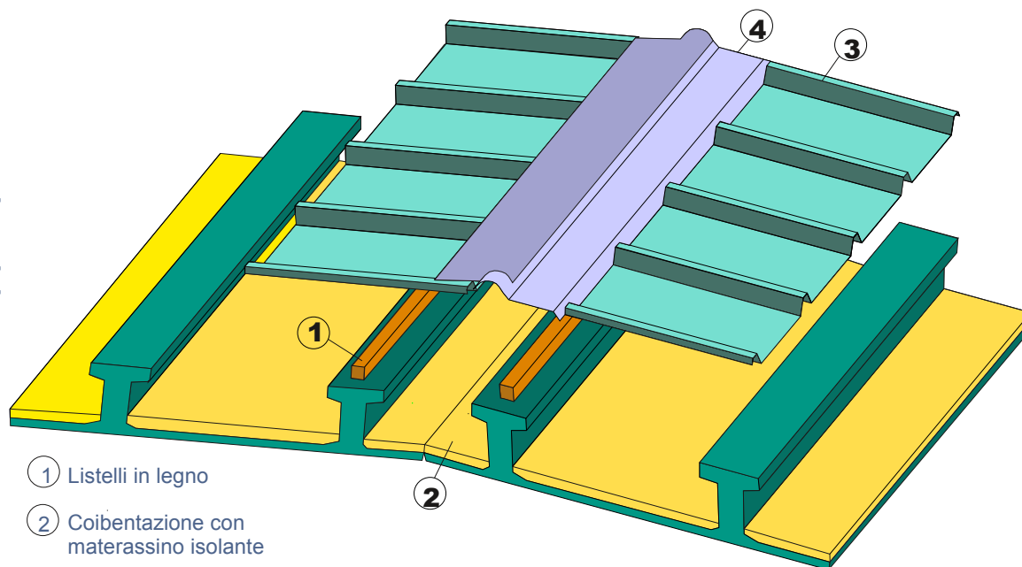
Particolare colmo
