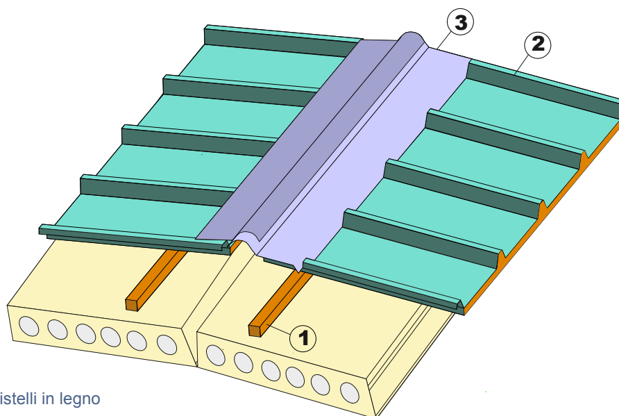
Particolare colmo
