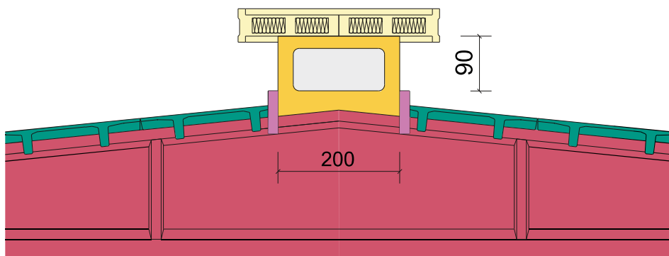
stralcio sezione trave doppia pendenza con torino
